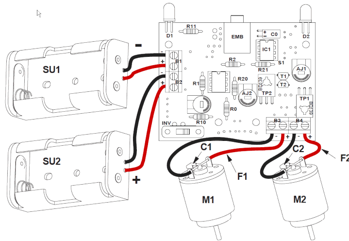
Carte programmable pour pilotage de 2 moteurs
